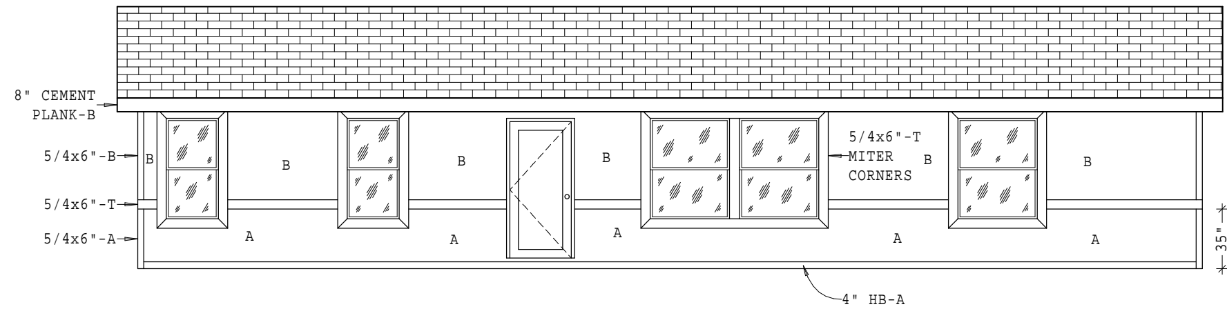
DOOR SIDE ELEVATION
